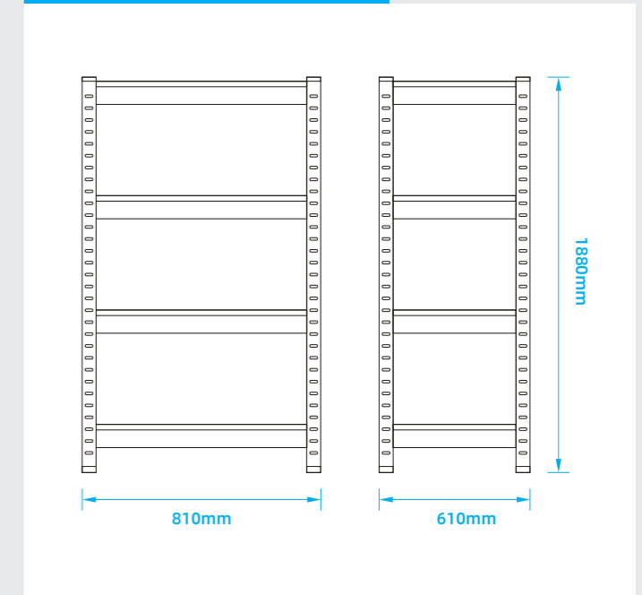
外型尺寸 Dimensions(Unit:mm)
