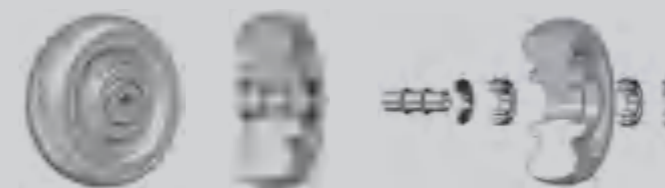
单轮剖视 双轴承工程共聚轮
