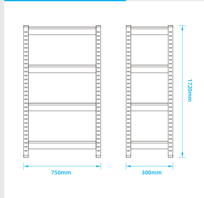
外型尺寸 Dimensions(Unit:mm)
